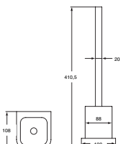
Bürstengarnitur 100 x 108 x 410,5 mm Modell N 1150 xx*
