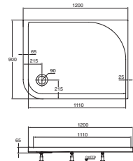
Brausewanne Rechteck Soft-Edge 1200 x 900 x 65 mm Version rechts Modell K 6184 01
