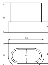
Zahnbecher 99 x 62 x 83 mm Modell N 1145 xx*
