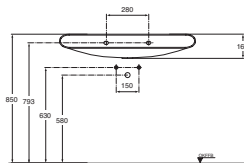
Wandsäule für Waschtisch Modell K 0074 xx*
