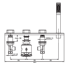
Bade-4-Loch-Armatur Modell A 3920 xx*
