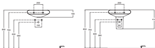
Wandsäule für Handwaschbecken Modell K 0076 xx*
