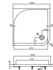
Brausewanne Quadrat Soft-Edge 1000 x 1000 x 65 mm Modell K 6181 01
