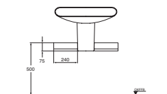
Wandsäulenablage kurz Echtholz furnier Eiche hell 240 x 75 x 140 mm Modell K 2195 xx*
