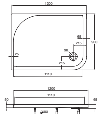
Brausewanne Rechteck Soft-Edge 1200 x 900 x 65 mm Version links Modell K 6185 01
