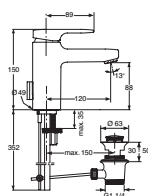
Waschtischarmatur Piccolo Ausladung 93 mm Auslaufhöhe 88 mm Modell A 3906 xx*
