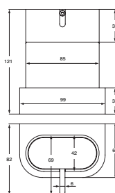
Lotionspender 99 x 82 x 121 mm Modell N 1146 xx*
