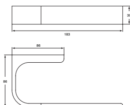
Reserverollenhalter 183 x 86 x 30 mm Modell N 1149 xx*
