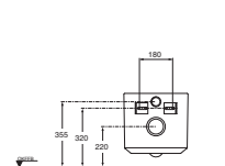
Wandbidet mit verdeckter Befestigung 345x580x330 mm Modell K 5053 xx*
