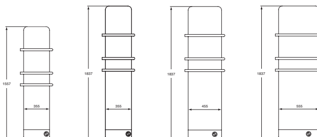
Heizkörper ca. 750 Watt mit elektrischer Zuheizung 555 x 1837 mm Modell K 2208 AC
