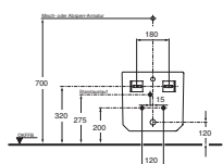
Standtiefspülklosett Kombination 350x640x835 mm Modell K 3114 xx*
