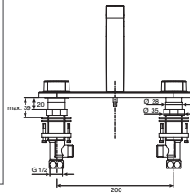
Waschtisch-3-Loch-Armatur Ausladung 154 mm Auslaufhöhe 136 Modell A 3907 xx*
