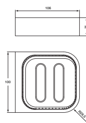
Seifenschale 100 x 106 x 30 mm Modell N 1147 xx*
