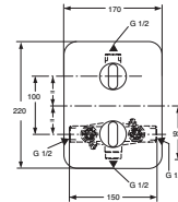
Bade-4-Loch-Armatur Modell A 3920 xx*
