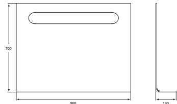
Spiegel 90 cm mit Licht und Ablage 900 x 160 x 700 mm Modell N 1152 AA
