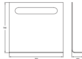
Spiegel 75 cm mit Licht und Ablage 750 x 160 x 700 mm Modell N 1153 AA
