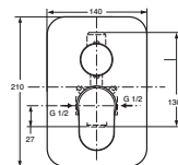
Einzel-Thermostat für Wandeinbau Modell A 3918 xx*
