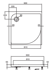
Brausewanne Quadrat 900 x 900 x 65 mm Modell K 6182 01
