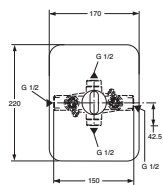
Badearmatur AP Aufputz Ausladung 165 mm Modell A 3914 xx*
