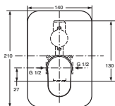
Zentral-Thermostat für Wandeinbau Modell A 3919 xx*
