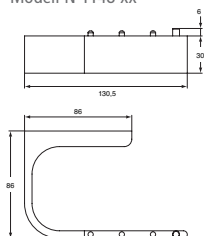
Papierrollenhalter 130,5 x 86 x 30 mm Modell N 1148 xx*
